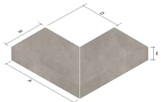
Schenkelplatte-Außenecke
